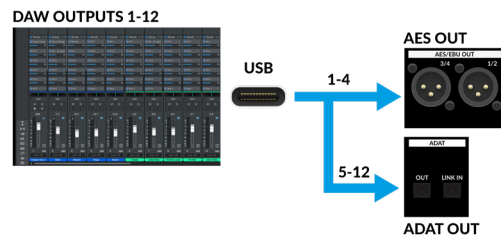
DAW はデジタル出力モードを供給: USB から供給される AES と ADAT。例: 44.1/48 kHz
