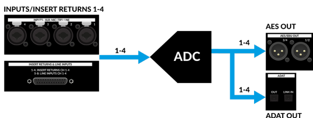
通常モード: A-D コンバーターから供給される AES と ADAT 出力
